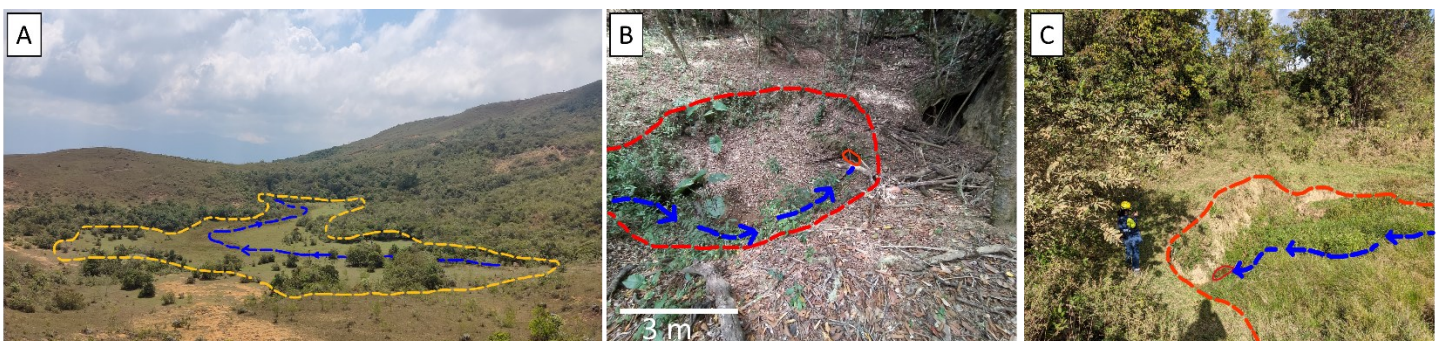
Fig. 6. A) Valle ciego con flujo de agua activo. B) y C) Sumideros de origen cárstico con flujo de agua activo. Fotografías: Los autores.
