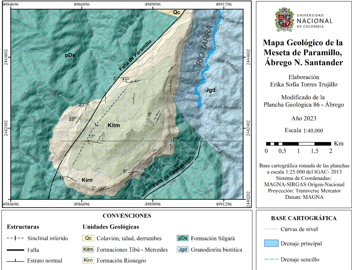
Fig. 2. Geología regional de la zona de estudio en la meseta de Paramillo donde se destaca la Formación Tibú - Mercedes en la cual se desarrolla el sistema cárstico. Fuente: modificado de Vargas y Arias (1981).
