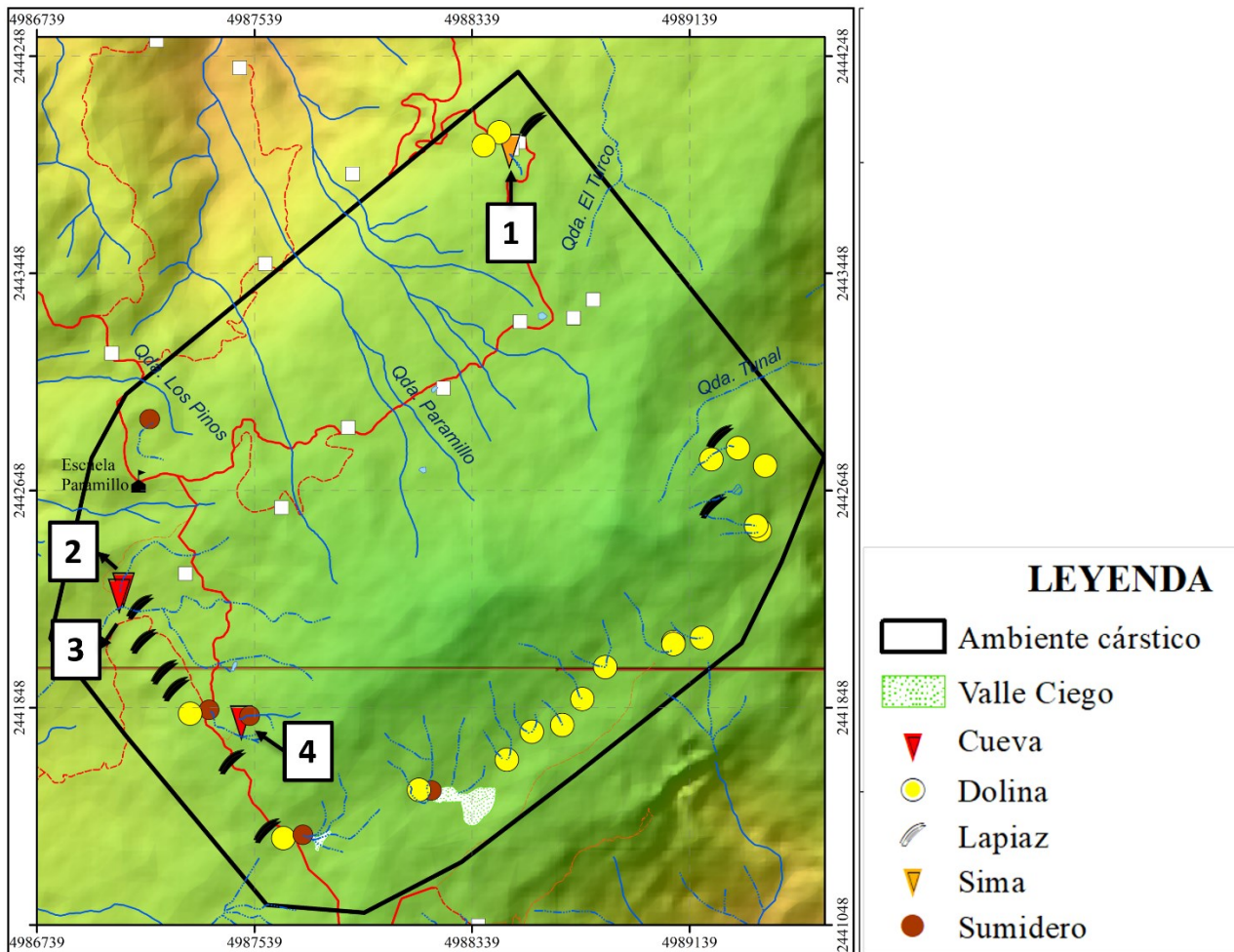
Fig. 7. Ubicación de las cuevas y sima en el área de estudio. 1. Sima Los Murciélagos, 2. Cueva La Chácara, 3. Cueva La Capilla, 4. Cueva Los Cedros.
