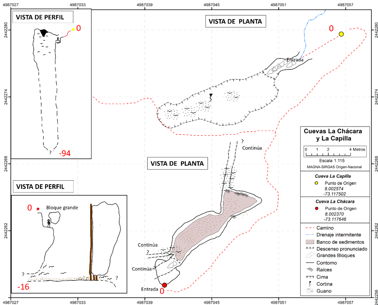
Fig. 11. Mapa espeleológico de las cuevas la Capilla y la Chácara. Arriba: Cueva la Capilla. Abajo: Cueva la Chácara. Nótese la poca distancia entre las cuevas.
