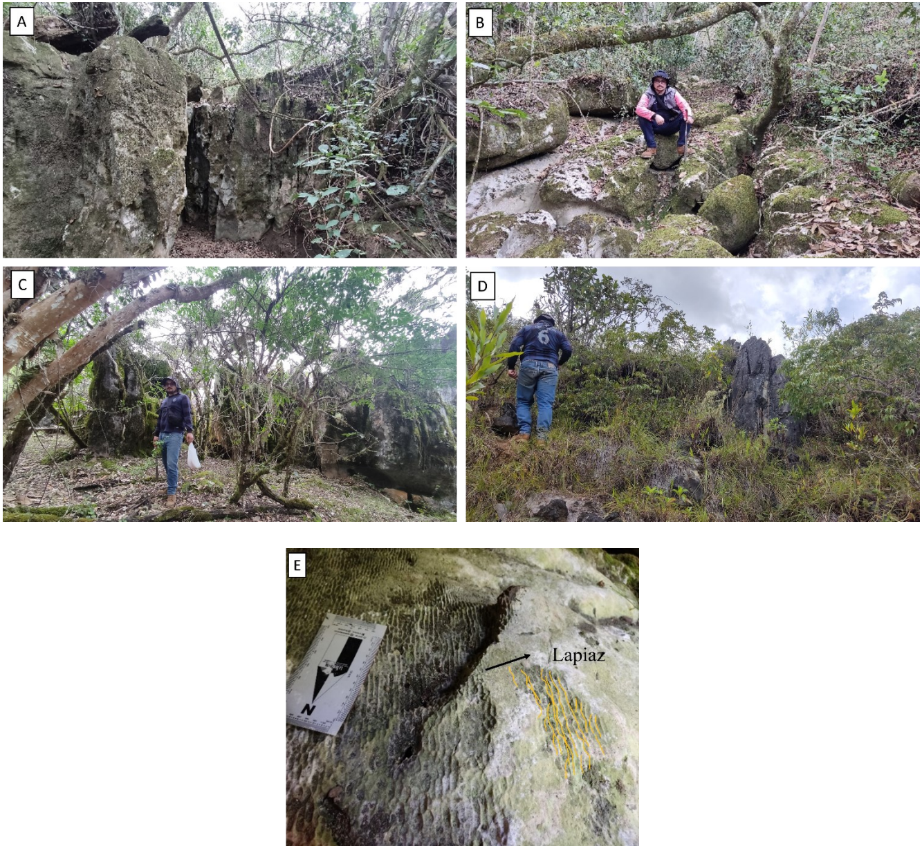
Fig. 5. A y B) Lapiaz tipo Kluftkarren. con formas suavizadas desarrollados a lo largo del drenaje. C y D) Lapiaz tipo Kluftkarren con formas angulosas desarrollado por precipitación. E) Lapiaz tipo Rillenkarrren alineado en roca calcárea masiva por gotas de lluvia. Fotografías: Los autores.
