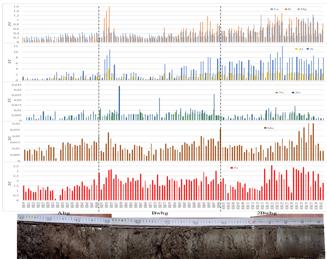
Figura 8. Paleosuelo clasificado como Typic Haplofibrists, de acuerdo con SSS (2022), localizado entre 19 y 144 cm del núcleo N14, extraído del Pantano la Bramadora, Sopetrán, Antioquia. En el N14 se analizaron, por fluorescencia de rayos X (FRX), todos los elementos, aunque, para el propósito de este artículo, solo se consideraron el Calcio (Ca), Potasio (K), Magnesio (Mg), Silicio (Si), Cinc (Zn), Níquel (Ni), Manganeso (Mn) y Hierro (Fe).
