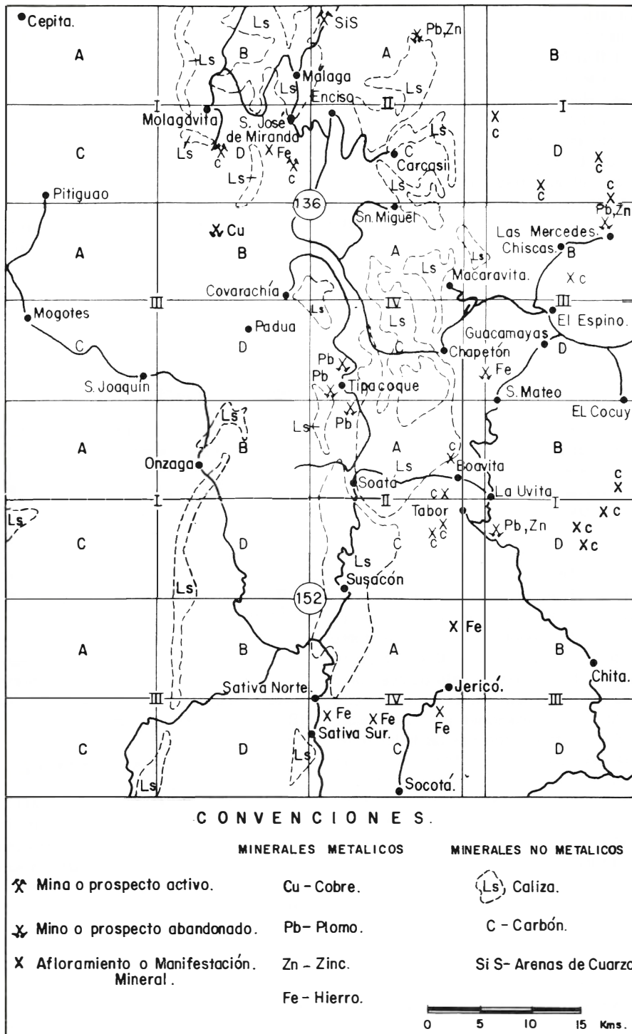
FIG. 2. Ocurrencias minerales del Cuadrángulo I-13
